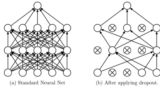
Hình 3. Mô hình mạng nơ-ron Drop. Bên trái: Một mạng nơ-ron tiêu chuẩn với 2 lớp hidden. Phải: Ví dụ về lưới mỏng được tạo ra bằng cách áp dụng tính năng dropout cho mạng ở bên trái. Các đơn vị bị gạch chéo đã bị loại bỏ [24]
